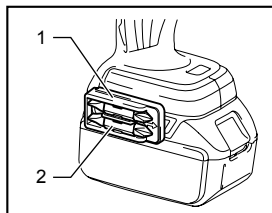
1. Porte-embout 2. Embout
