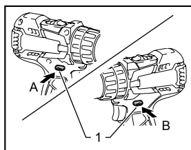
1. Levier inverseur
